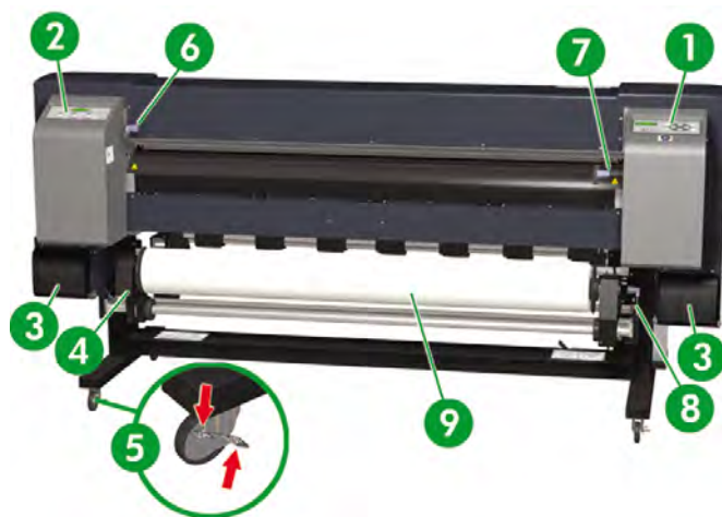
前視圖
