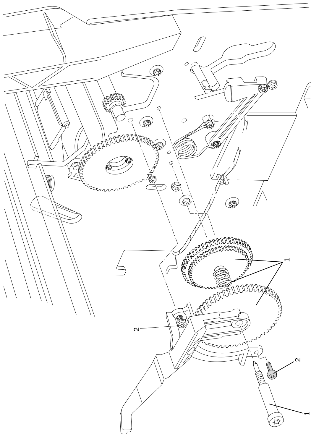
Figura 10: Conjunto de Engrenagens
