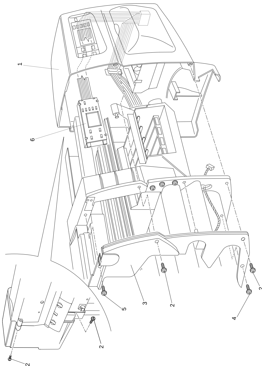
Figura 6: Tampa Direita
